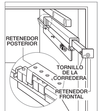
Ajuste horizontal.
